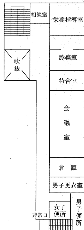
2 階
